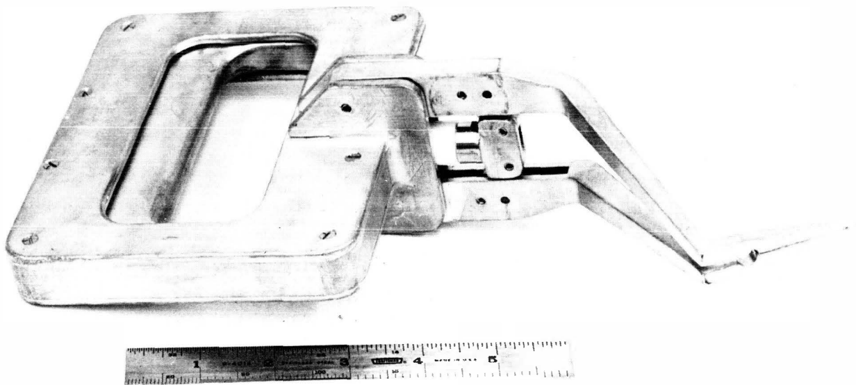
Figure 24.- Tweezers (SEZ 36104416-301).
