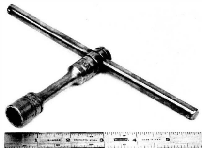
Figure 23.- T-handle (SEZ 36106104-301).
