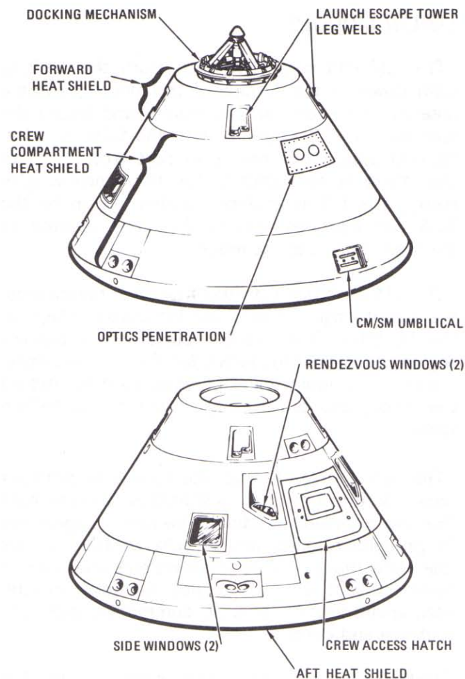
Command module
