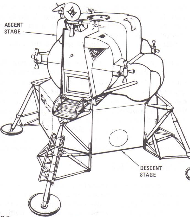
Lunar module
