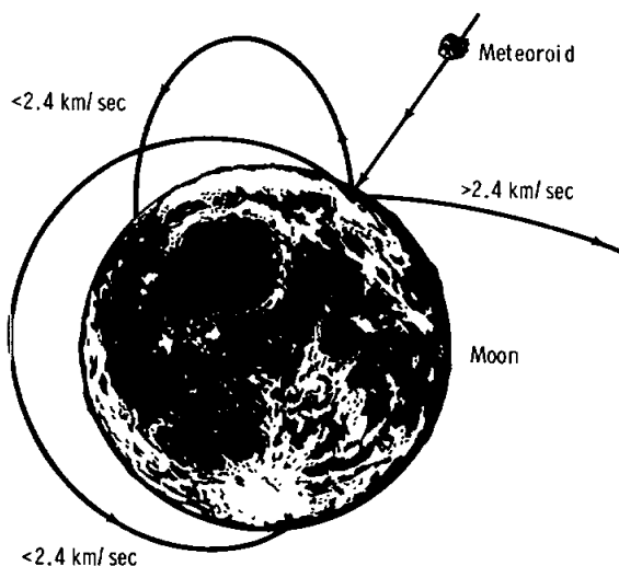
FIGURE 16-1.—Lunar ejecta.
