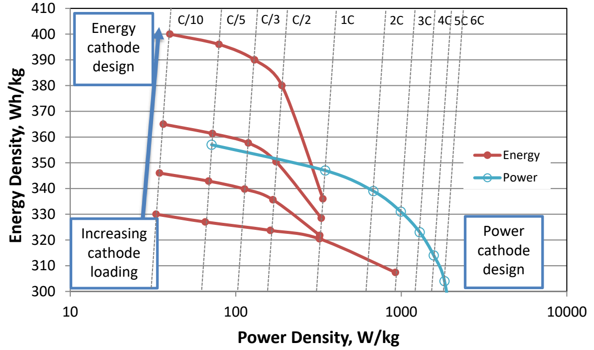
Si NW anode/LCO Ragone Plot
