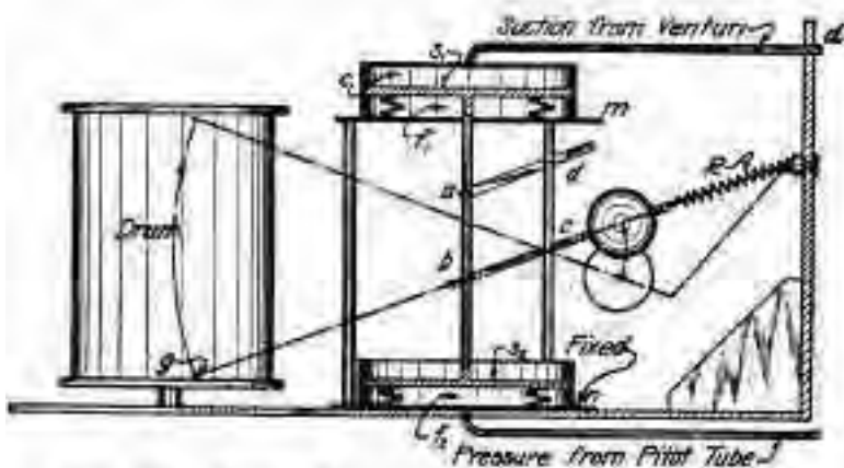
Fig. 13—Recording apparatus of Toussaint-Lepère air speed meter
