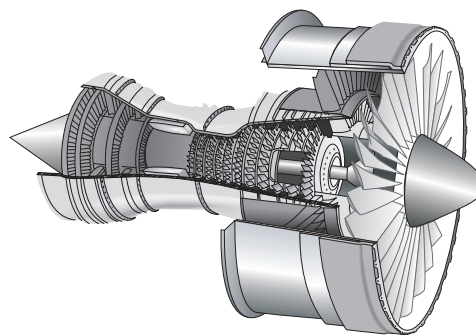
motor
