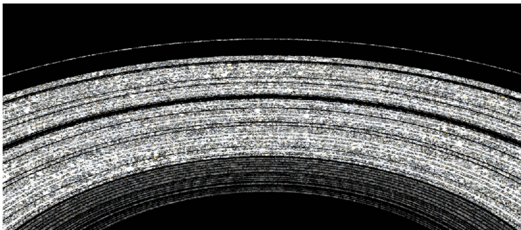
Huygens
